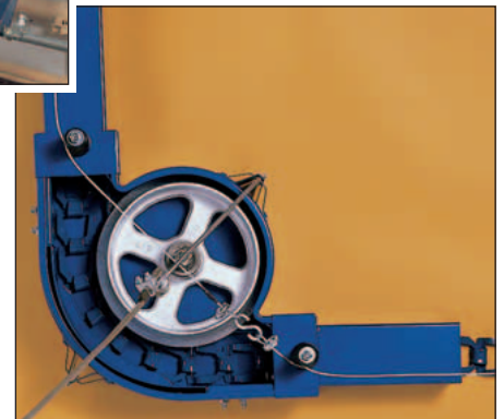
Autolimit silo scale
